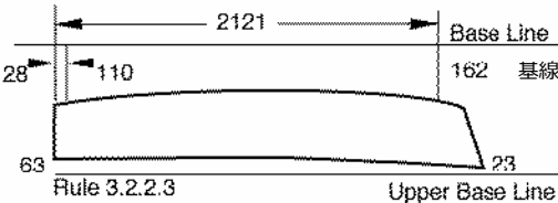
注：ノリは裏返しにされている。 Note: Hull is shown inverted
